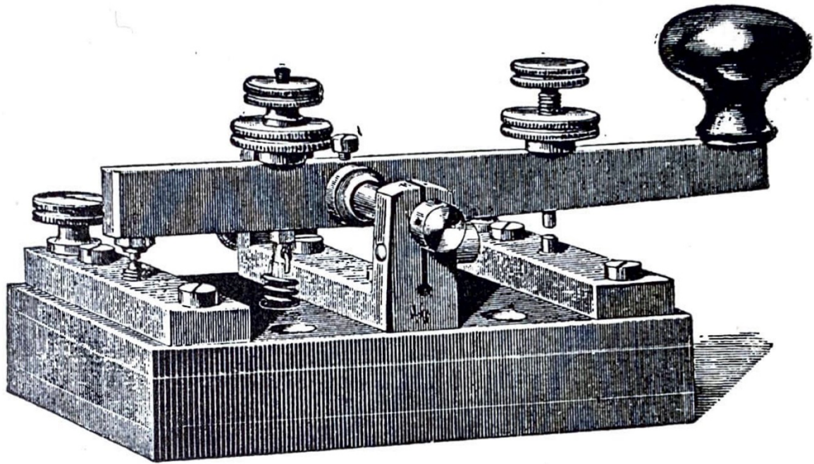
562. Der Morse-Taster.
